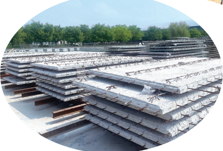
工厂的预制墙板。
