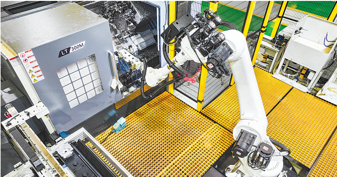
这是二〇二五年五月九日在位于重庆市北碚区的重庆顺多利机车有限公司精工基地拍摄的自动化生产作业现场(无人机照片)。新华社发
