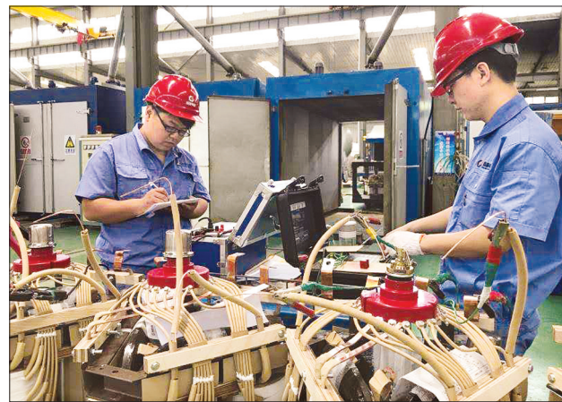
近日,在位于永年区工业园区内的河北高晶电器设备有限公司,工人正在对生产的变压器进行参数检测。该公司S13型110kV三相油浸式立体卷铁心电力变压器的产品标准已转化为我省地方标准。 赵明 摄
