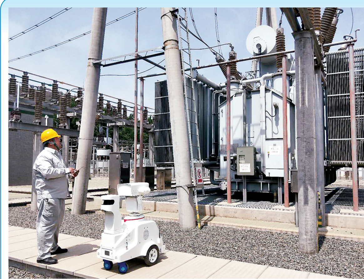
5月9日,承德供电公司员工马利在220千伏线路送电后利用智能机器人在220千伏潮河变电站对1号主变进行检测。截至目前,该公司变电运维室所辖变电站智能巡检机器人已投运4台,共巡视800余次,全部运行正常。变电智能机器人的投运,有效提高了设备巡视质量,提升了运维效率,为变电站顺利实现无人值班,确保设备安全运行提供了强有力的保障。徐娜 王冰洋 摄
